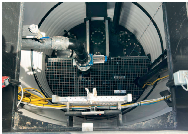
Przepompownia ścieków – tłocznia w Mrokowie.
