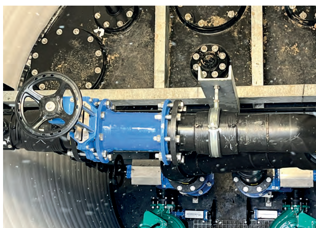
Przepompownia ścieków – tłocznia P11 we Władysławowie.
