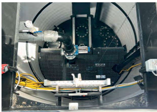
Przepompownia ścieków – tłocznia w Mrokwie.
